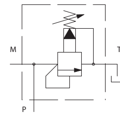
Schaltplan 2
