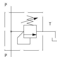
Schaltplan 1
